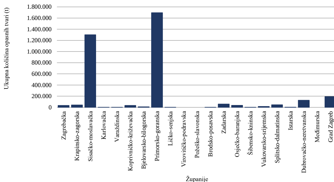
Slika 6. Ukupna količina opasnih tvari (t) u područjima postrojenja višeg i nižeg razreda u RH, po županijama u 2020. godini
