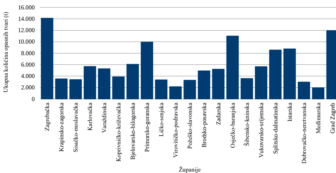
Slika 11. Prikaz ukupnih količina prijavljenih opasnih tvari (t) obveznika Priloga II.A Uredbe u RPOT/OPVN po županijama, u 2020. godini u RH
