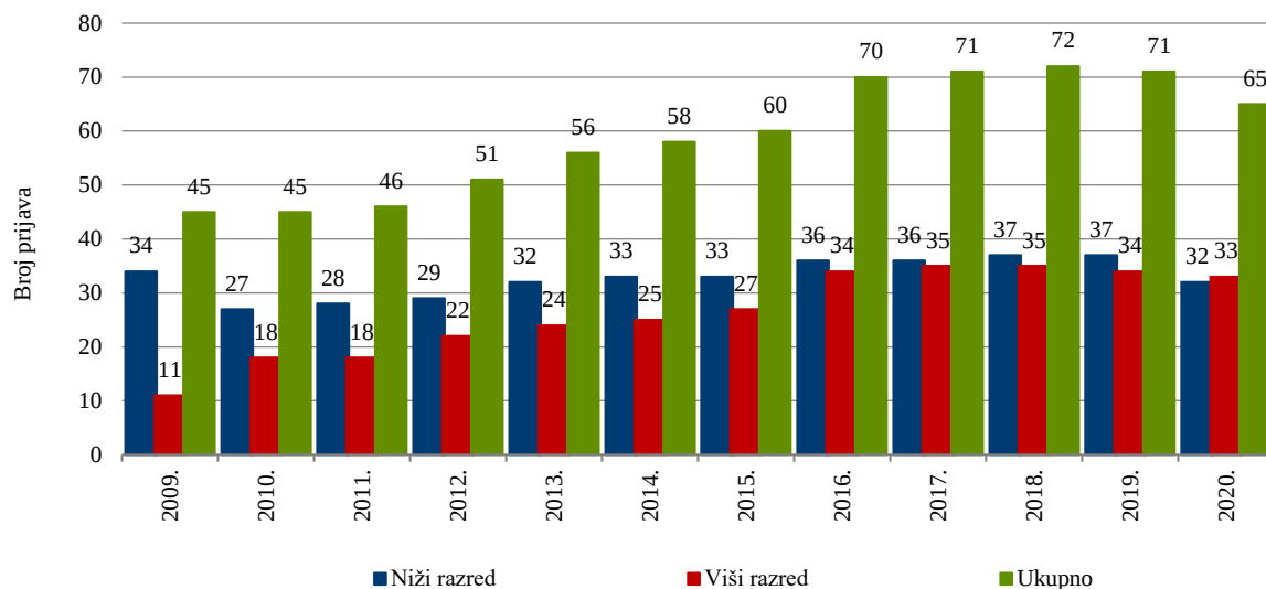
Slika 2. Prikaz trenda prijave područja postrojenja višeg i nižeg razreda od 2009. do 2020. godine u RH
