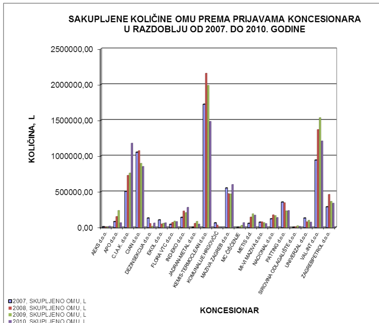
Graf 1. Usporedba sakupljenih količina otpadnih mazivih ulja prema prijavama koncesionara u razdoblju od 2007. do 2010. godine
