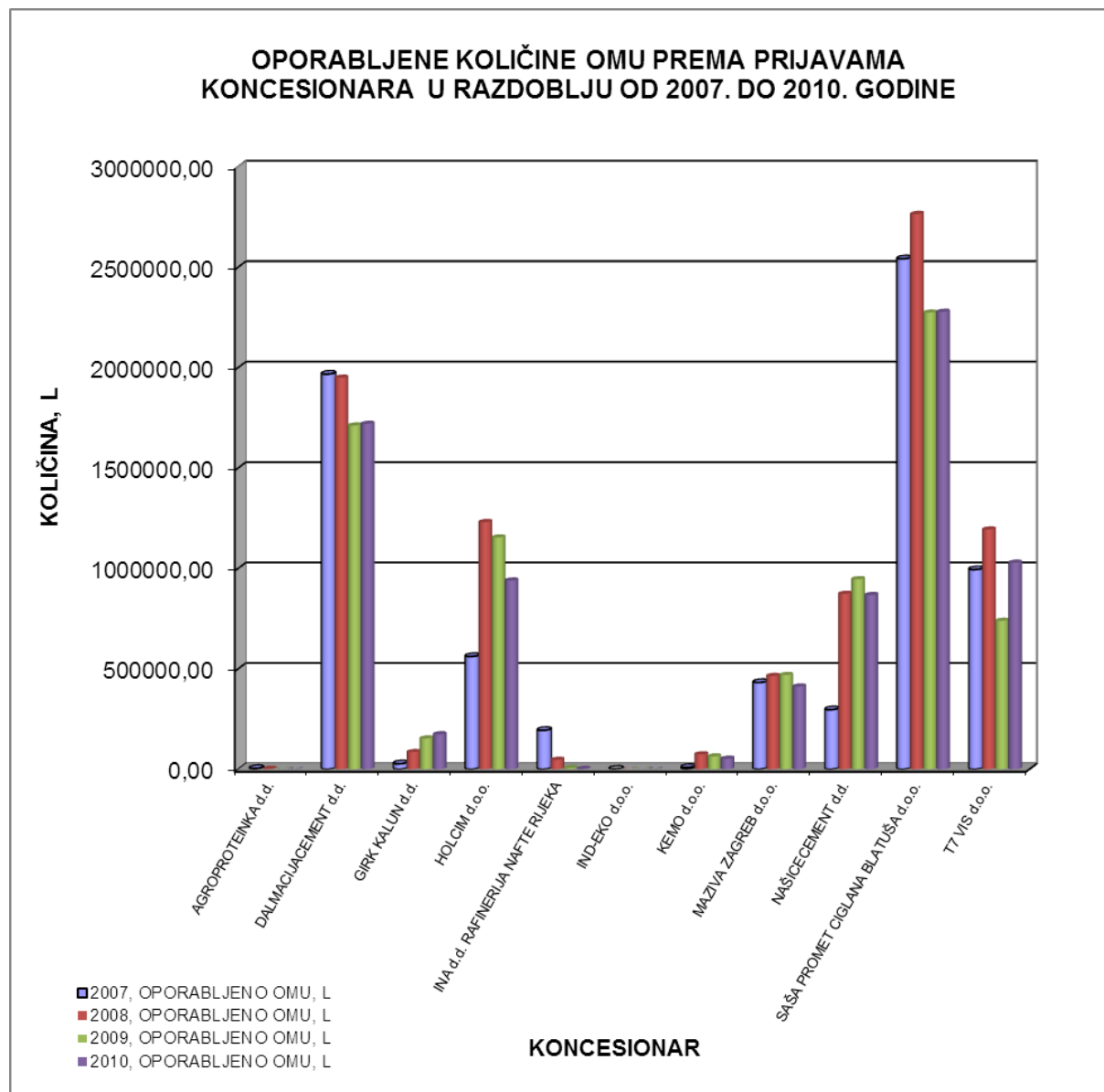
Graf 3. Usporedba oporabljenih količina otpadnih mazivih ulja prema prijavama koncesionara u razdoblju od 2007. do 2010. godine
