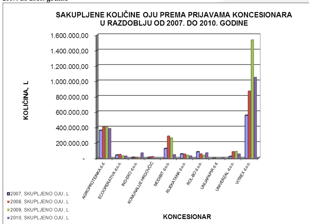
Graf 2. Usporedba sakupljenih količina otpadnih jestivih ulja prema prijavama koncesionara u razdoblju od 2007. do 2010. godine
