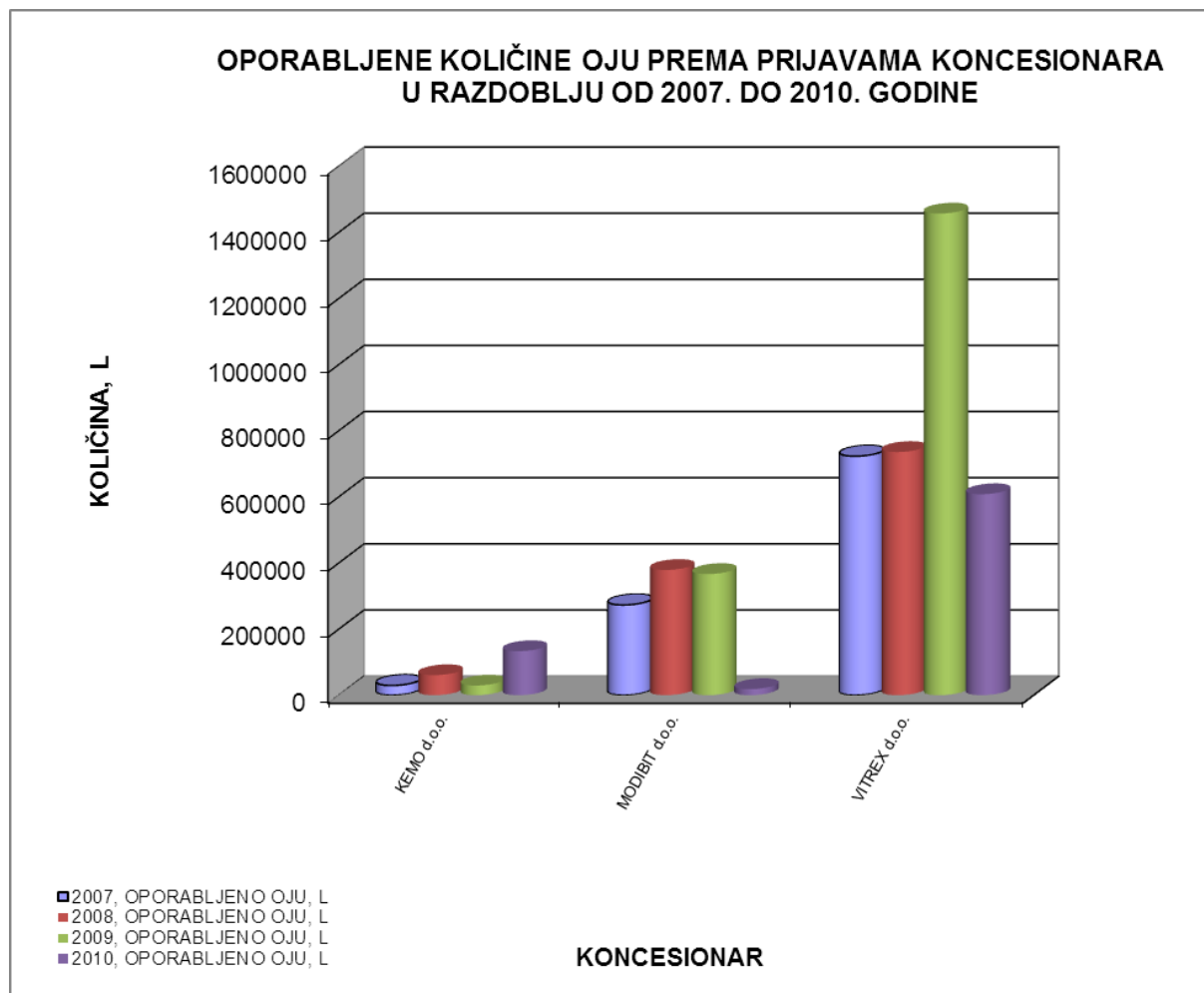
Graf 4. Usporedba oporabljenih količina otpadnih jestivih ulja prema prijavama koncesionara u razdoblju od 2007. do 2010. godine
